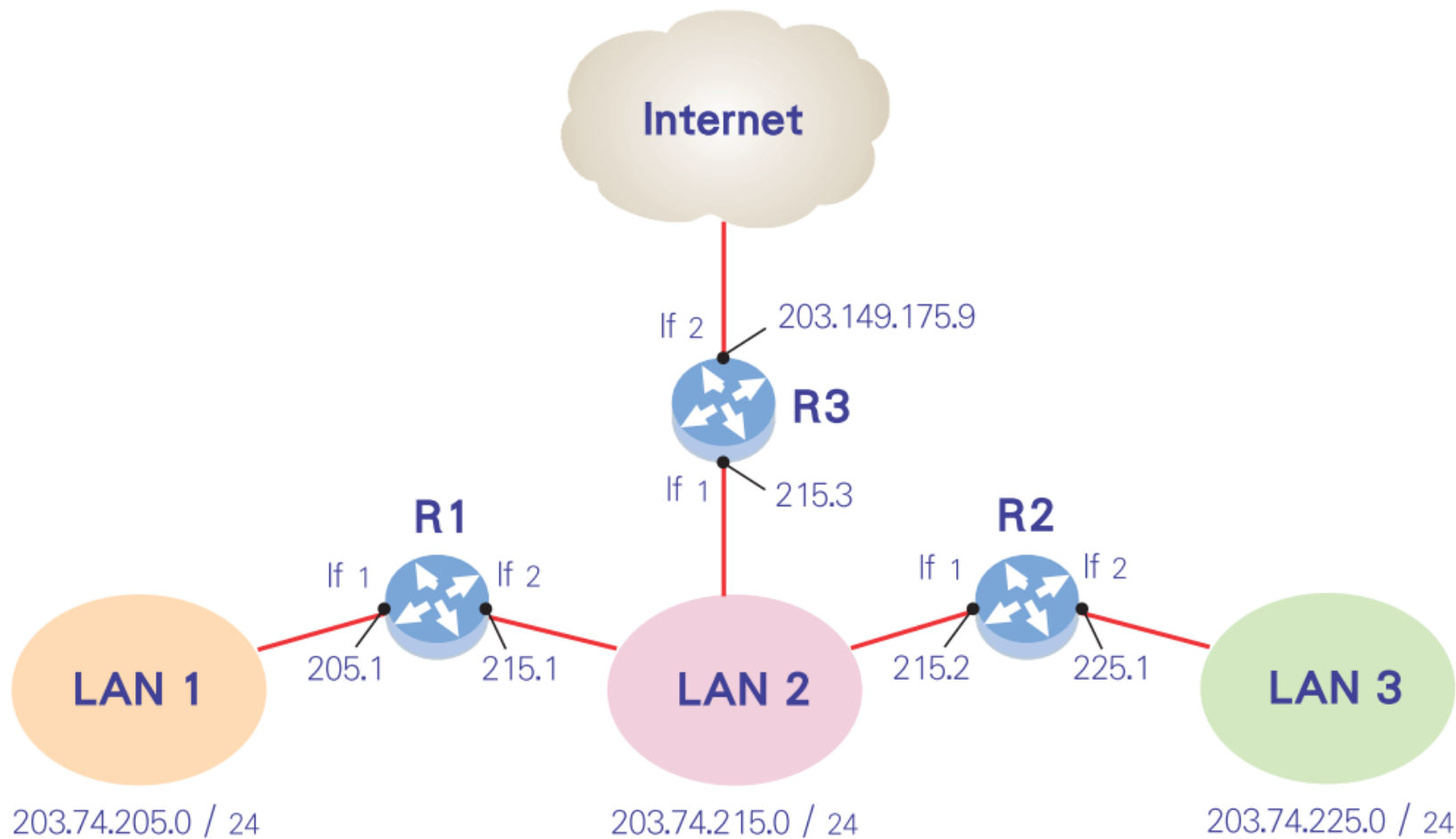
圖 9-7 2 部路由器 + 預設路由的網路
